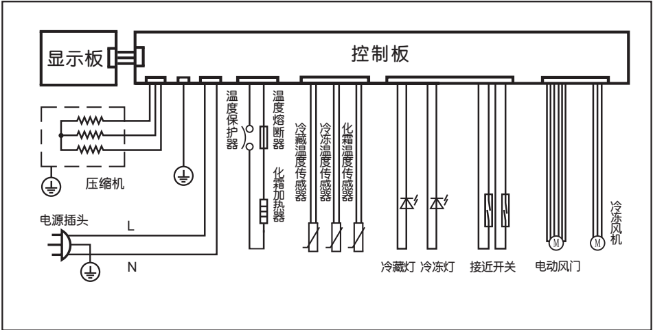
电路图
