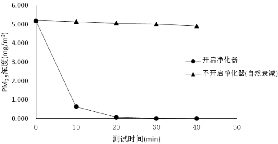
PM 2.5 衰减曲线
