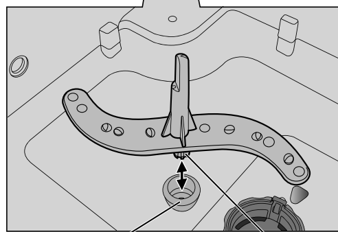
机体的管道部分 喷嘴的管道部分
