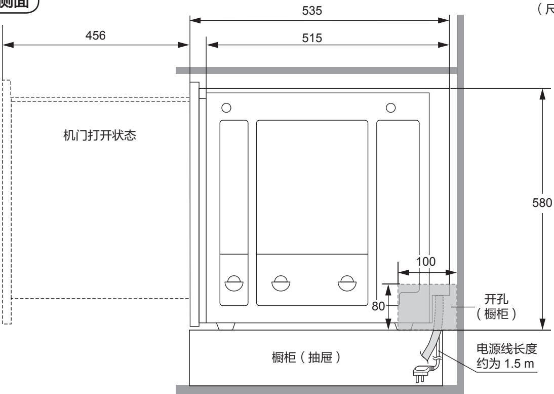
机体侧面
