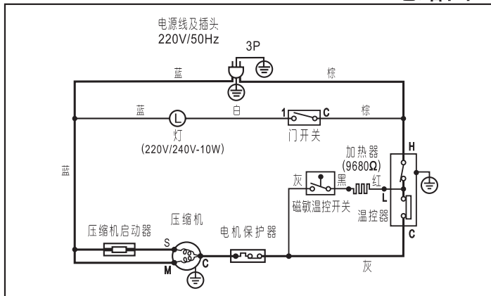
NR-B17S6/NR-B18S6/NR-B19S6电路图
