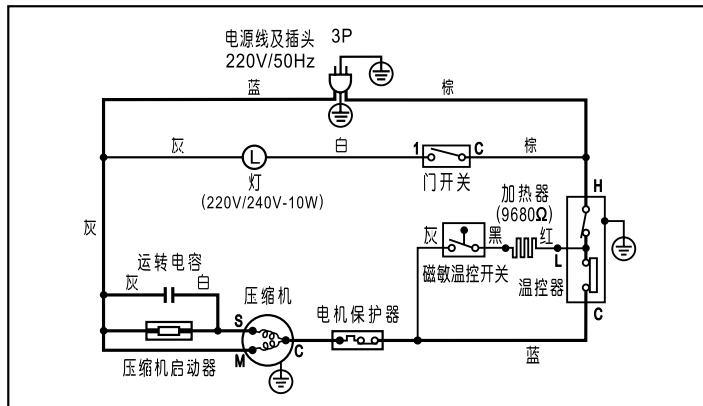
NR-B17S7/NR-B18S7/NR-B19S7 电路图
