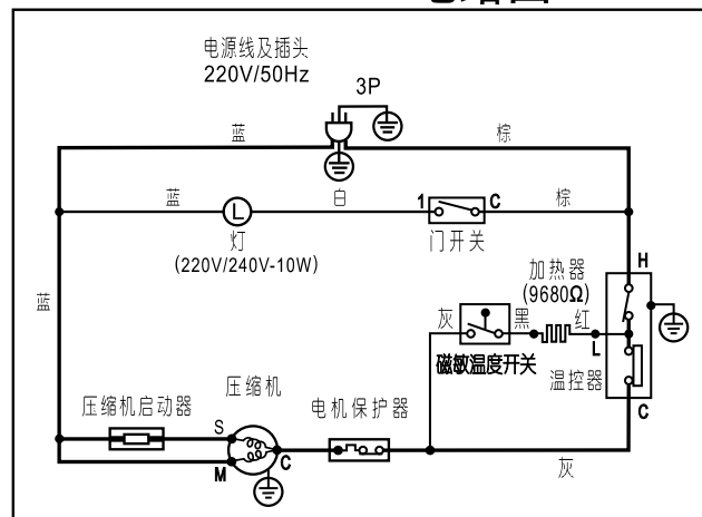
NR-B21S7电路图
