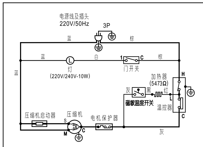
NR-B23S7电路图
