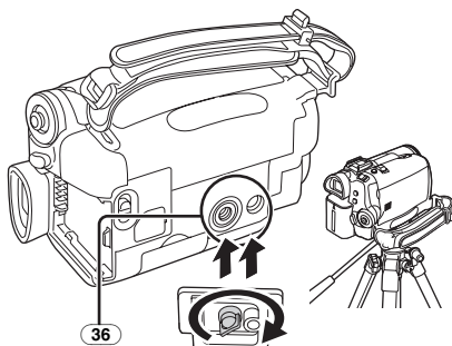
36 三脚架插座
