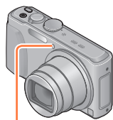
AF辅助灯
